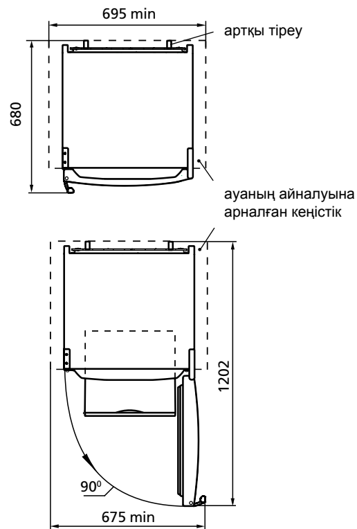
2 сурет — Тоңазытқыш (жоғарыдан көрініс)
