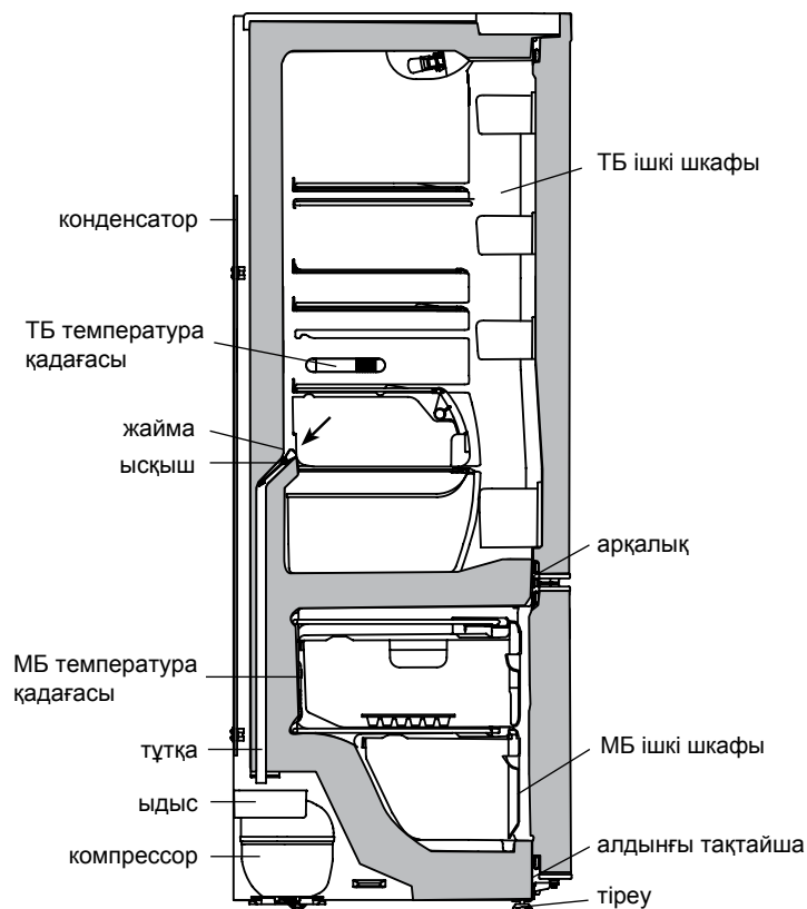
6 сурет — ТБ еріген судың ағылу сызбасы
