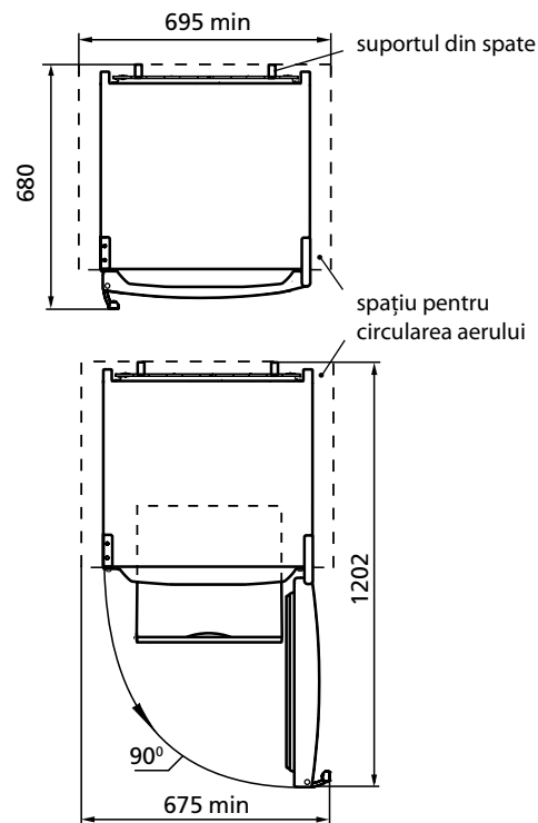
Figura 2 — Frigider (privire den sus)
