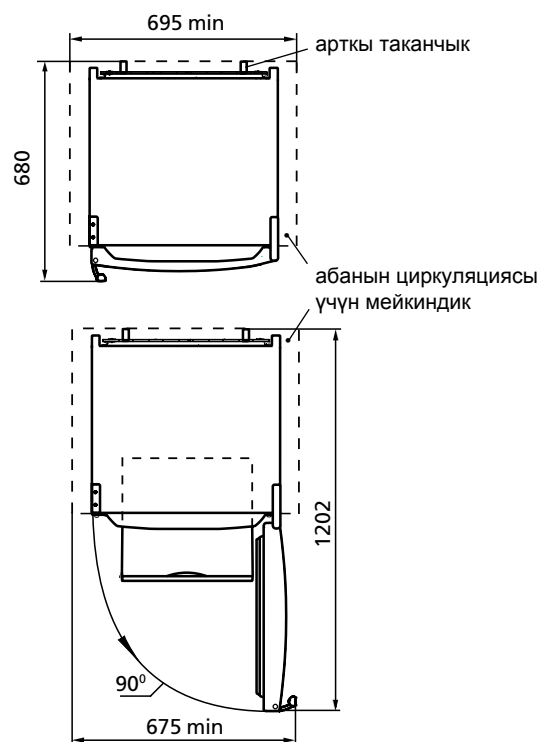
2-сүрөт — Муздаткыч (үстүнөн көрүнүшү)
