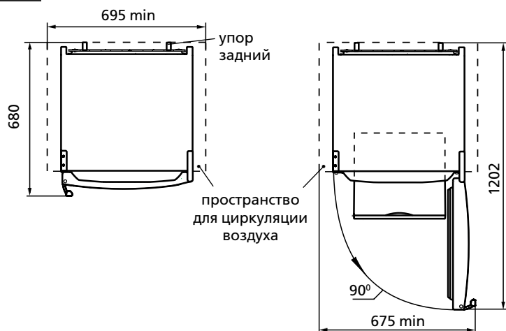
Рисунок 2 — Холодильник (вид сверху)
