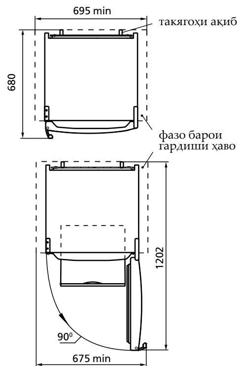
Расми 2 — Яхдон (намуди он аз қисми боло)
