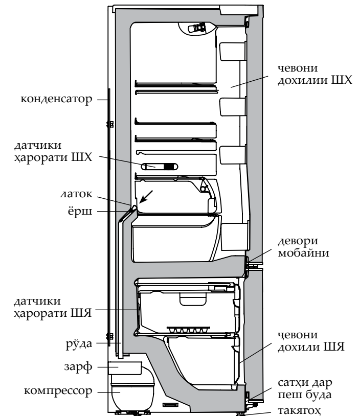
Расми 6 – Нақшаи рехтани об аз ШХ
