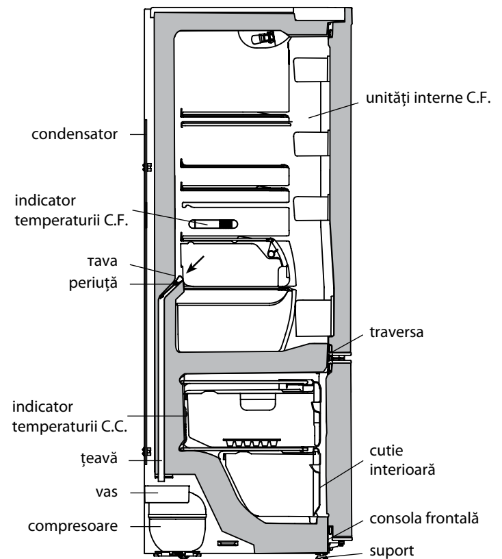
Figura 6 — Schemă de scurgere de apă topită din C.F.
