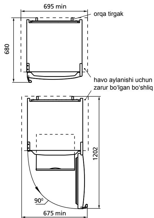
2 rasm — Sovutgich (tepadan ko'rinish)
