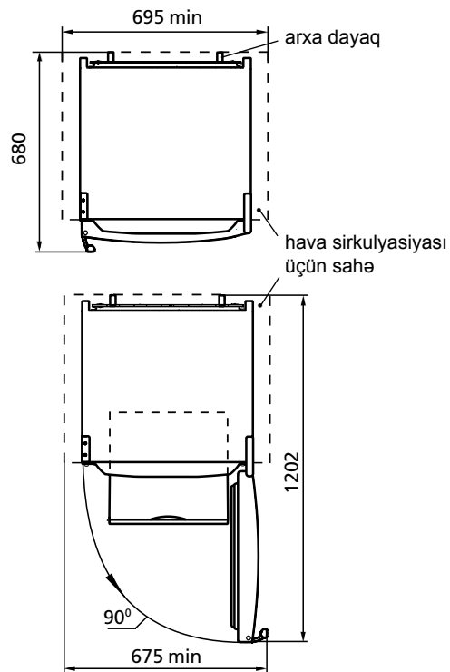
Rəsim 2 — Soyuducu (üstədən görünüşü)
