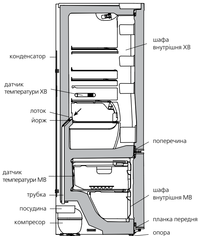
Рисунок 6 — Схема зливу талої води із ХВ
