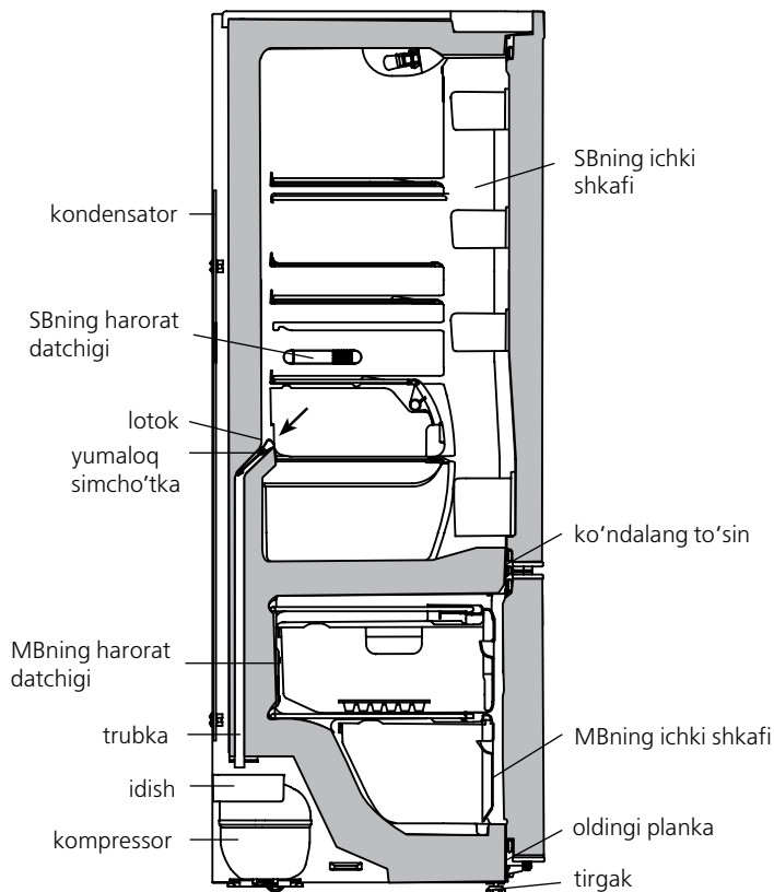
6 rasm — SBdan erigan suv oqib ketish sxemasi
