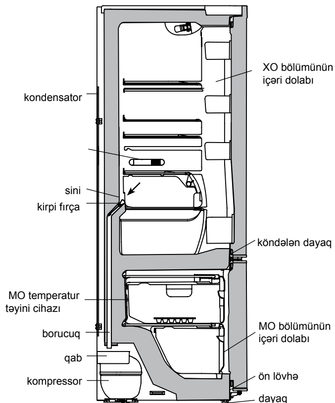
Rəsim 6 — XO bölümünün ərmiş axıntı sularının tökülməsi sxemi
